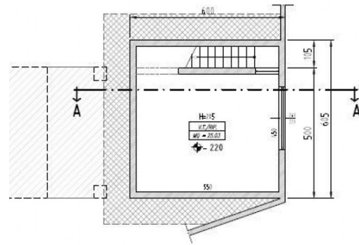
PIANTA PIANO SEMINTERRATO
