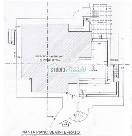
PIANTA PIANO SEMINTERRATO
